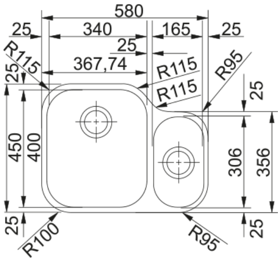
Мойка AMX 160, 580x450 мм, без крыла, нерж.сталь, 3 1/2", вентиль, короб
