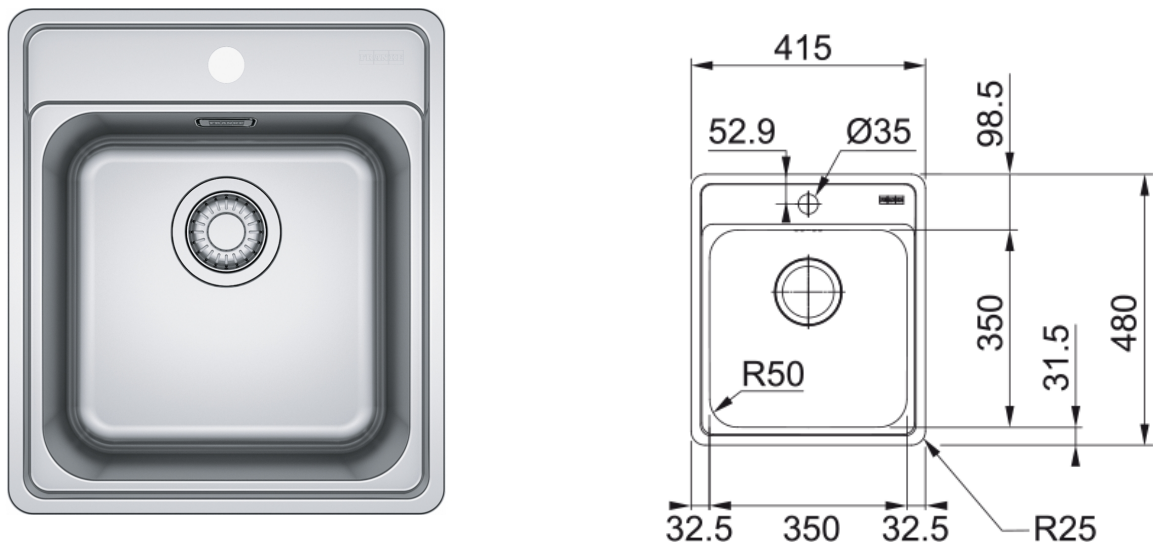
Мойка BCX 610-42, 415x480 мм, 3 1/2", нерж.сталь, без вентиля, перелив , отверстие под смеситель
