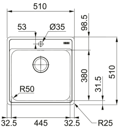
Мойка BCX 610-51, 510x510 мм, 3 1/2", нерж.сталь, без вентиля, перелив, отверстие под смеситель
