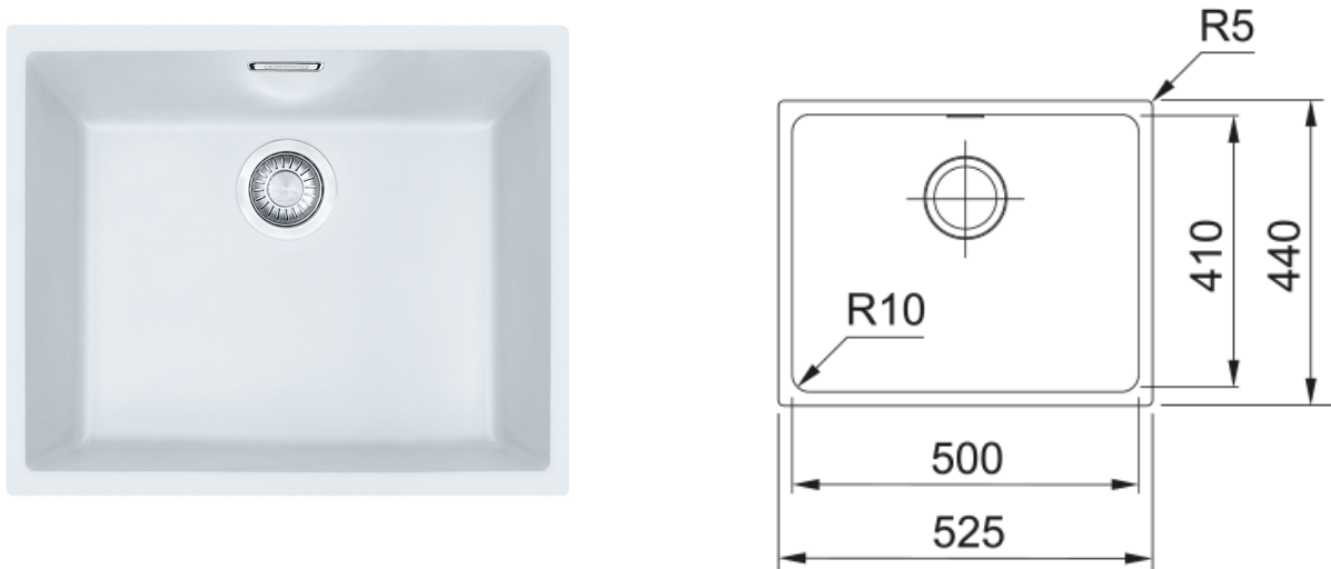
Мойка SID 110-50, 3 1/2", стоп-вентиль в комплекте, сифон, скрытый перелив в чаше
