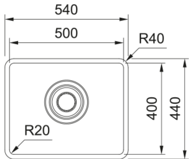
Мойка Maris Quiet MQX 110-50, полированная нержавеющая сталь, подстольный монтаж, 1 чаша без крыла, 500x400 мм.
