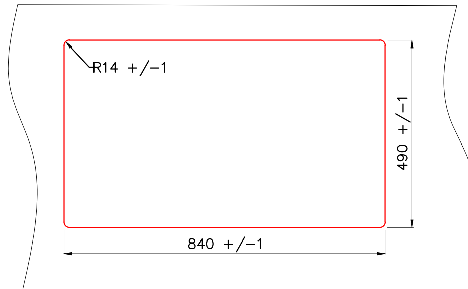
Врезной монтаж мойки (I)
